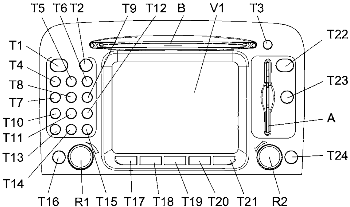
Fig. 1 Commandes du système CONNECT Nav+
